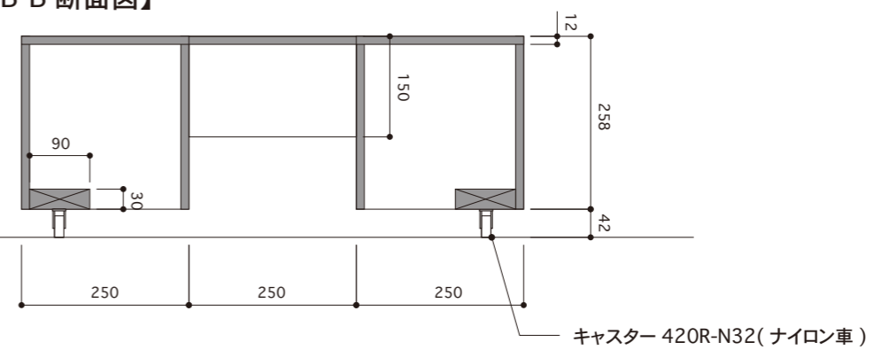
【B-B 断面図】
