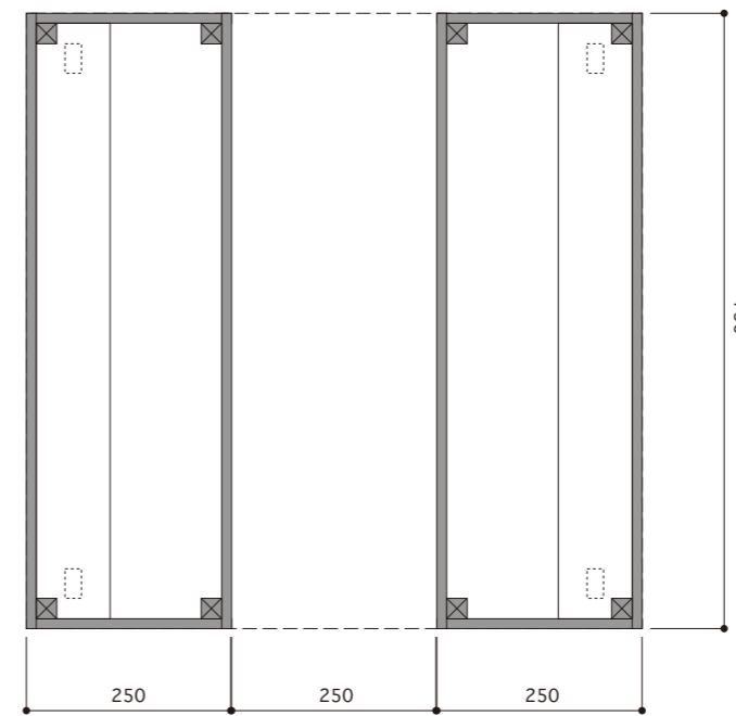
【A-A 断面図】
